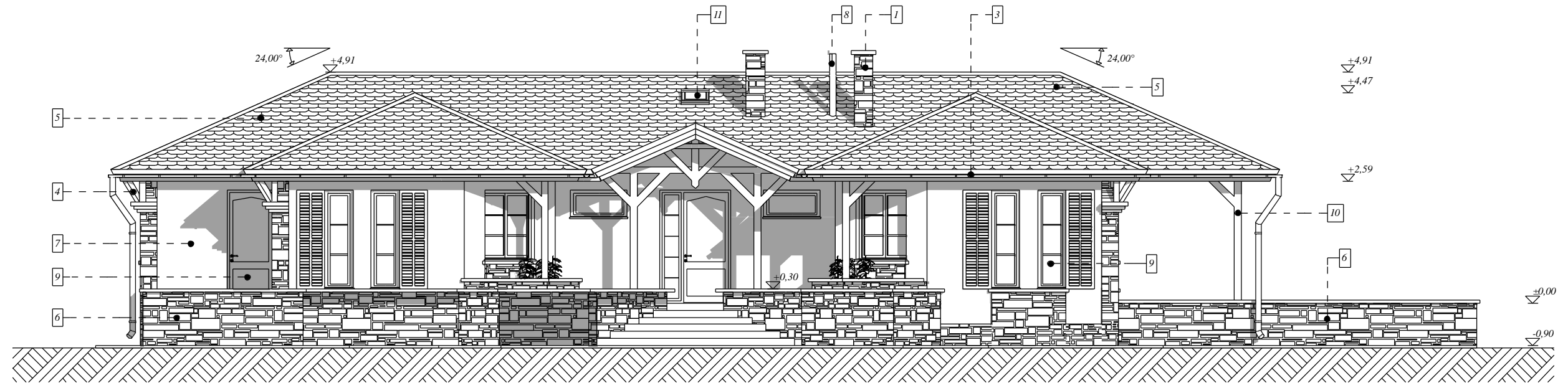
Déli homlokzat M=1:100
