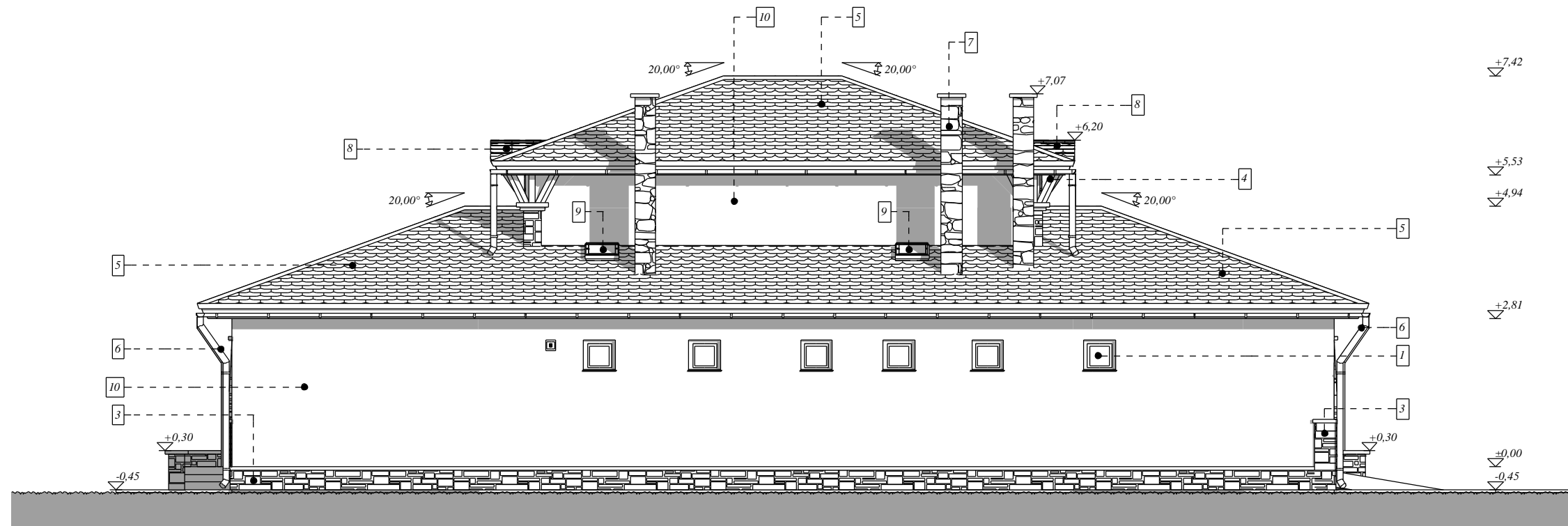
Északi Homlokzat M=1:100
